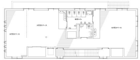
2階 平面図
